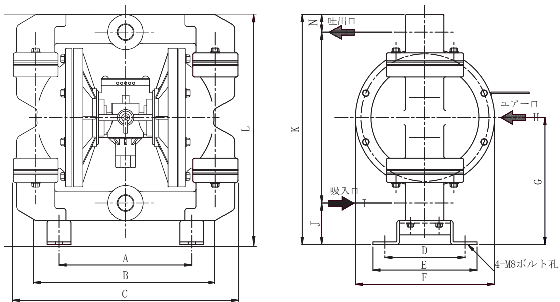
L型 (K6)
