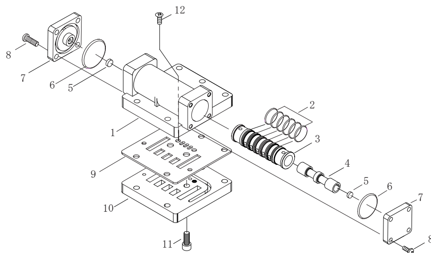
部品No.39 メインバルブ組
