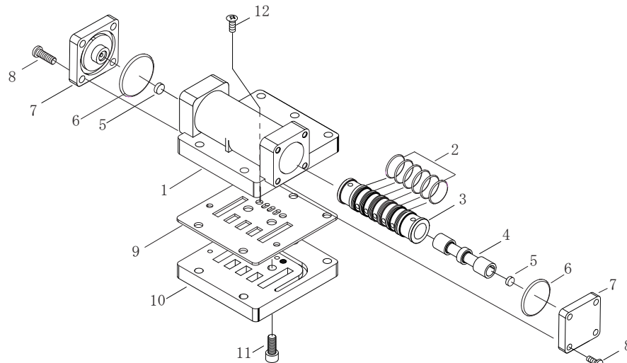
部品No.39 メインバルブ組
